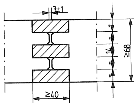
Schnitt K-K
