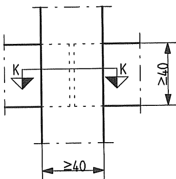
Ansicht Rahmen-Kreuz-Verbindung
