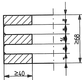
Schnitt I - I
