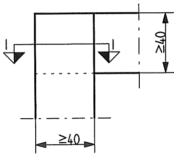
Ansicht Rahmen-Verbindung 90°
