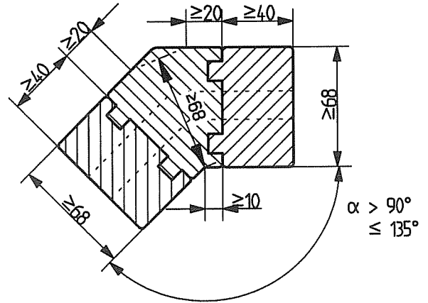
Schnitt F-F Variante: bei Ecke >90° und <135°
