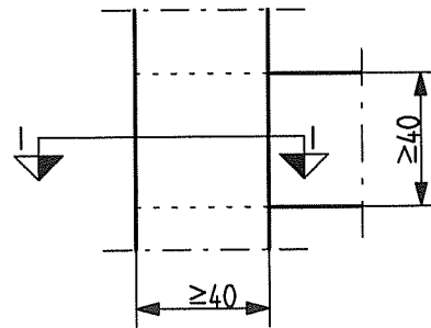
Ansicht Rahmen-T-Verbindung
