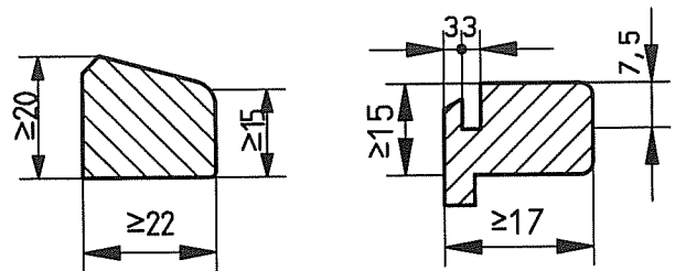
Glashalteleiste
