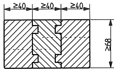
Schnitt E-E Variante: mit "Koppelholz"
