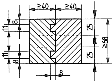
Schnitt D-D Längsverbinding
