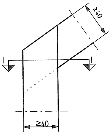
Ansicht Rahmen-Verbindung >90°
