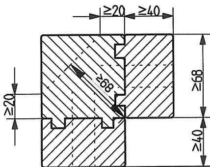
Schnitt F-F Variante: bei Ecke >135° und <180°
